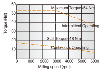
αiS 22/6000 (4.5 kW)
